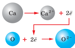
Рис. 7. Схема образования ионной связи между атомами кальция и кислорода
