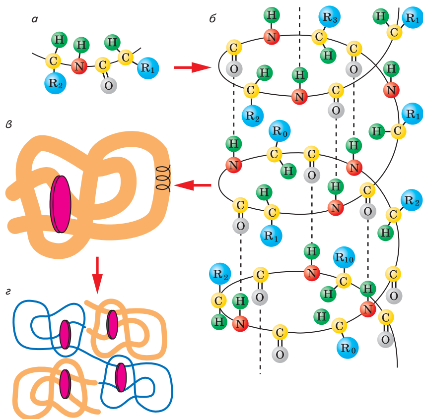
Рис. 46. Структура белковой молекулы, состоящей из нескольких полипептидных цепочек: a — первичная; b — вторичная; в — третичная; г — четвертичная
