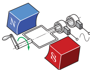
Рис. 137. Схема устройства электрического генератора
